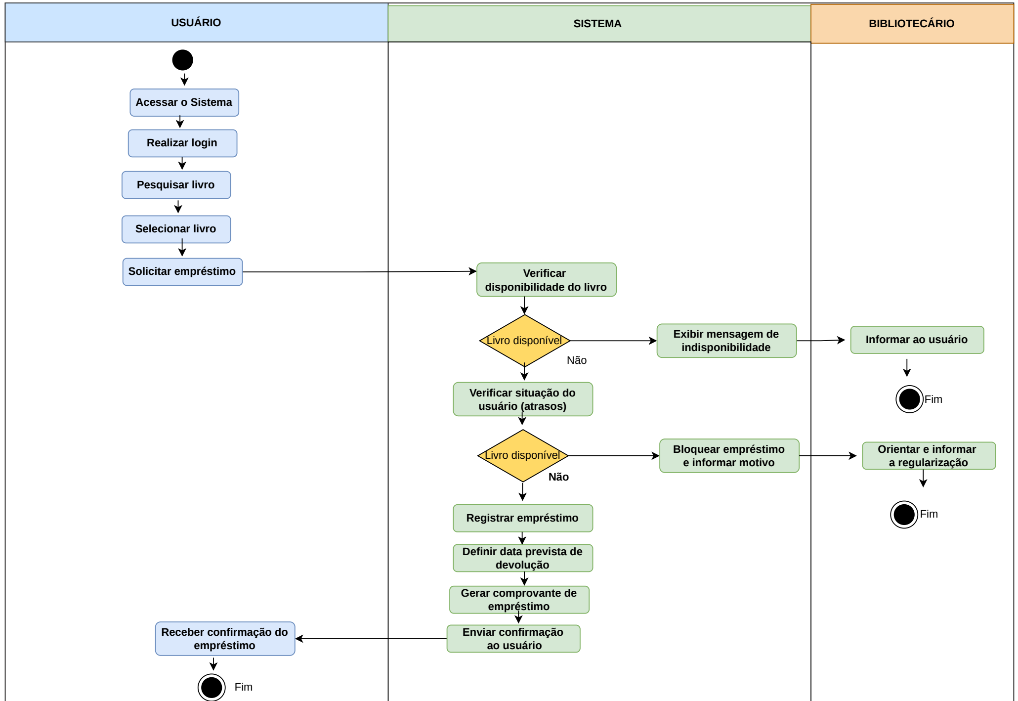
DIAGRAMA DE ATIVIDADES - REALIZAR EMPRÉSTIMOS
