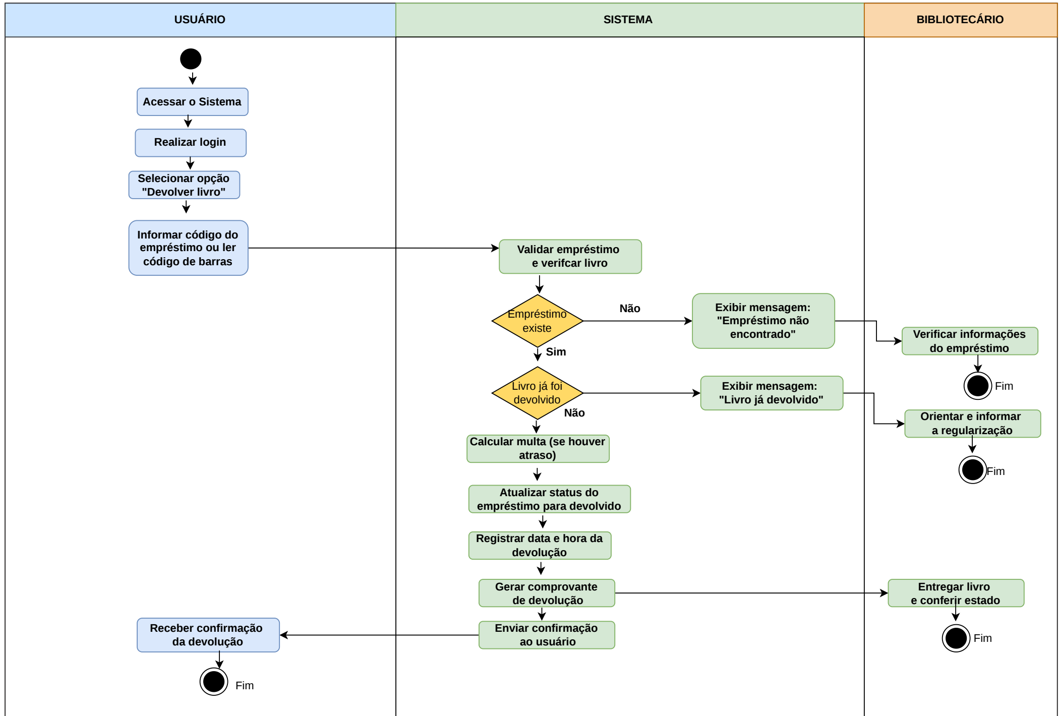
DIAGRAMA DE ATIVIDADES - PROCESSAR DEVOLUÇÃO DE LIVRO
